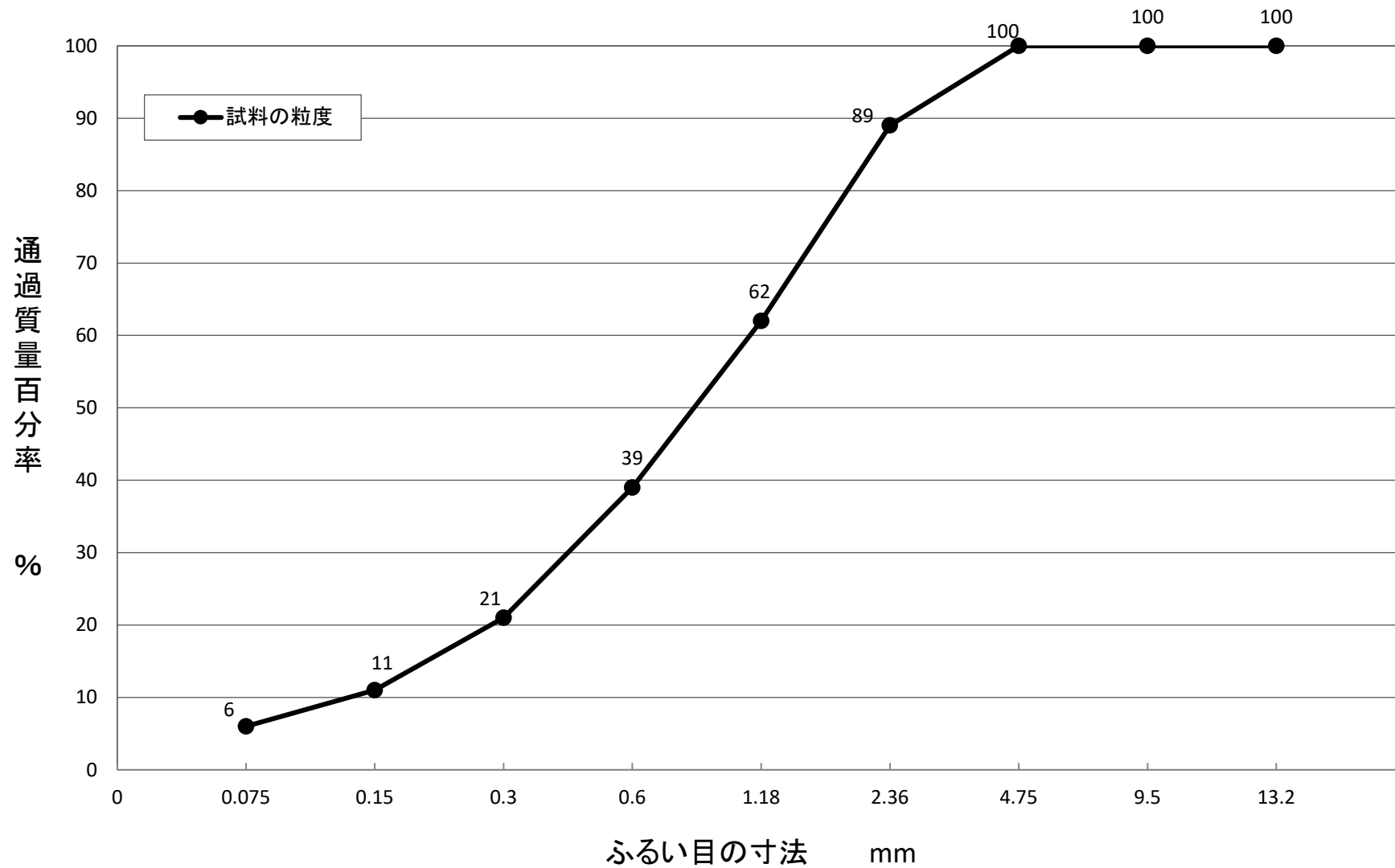
図—1 粒度試験結果
